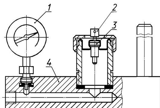
1 — манометр; 2 — головка с соплом; 3 — aerosольный клапан; 4 — основание приспособления
